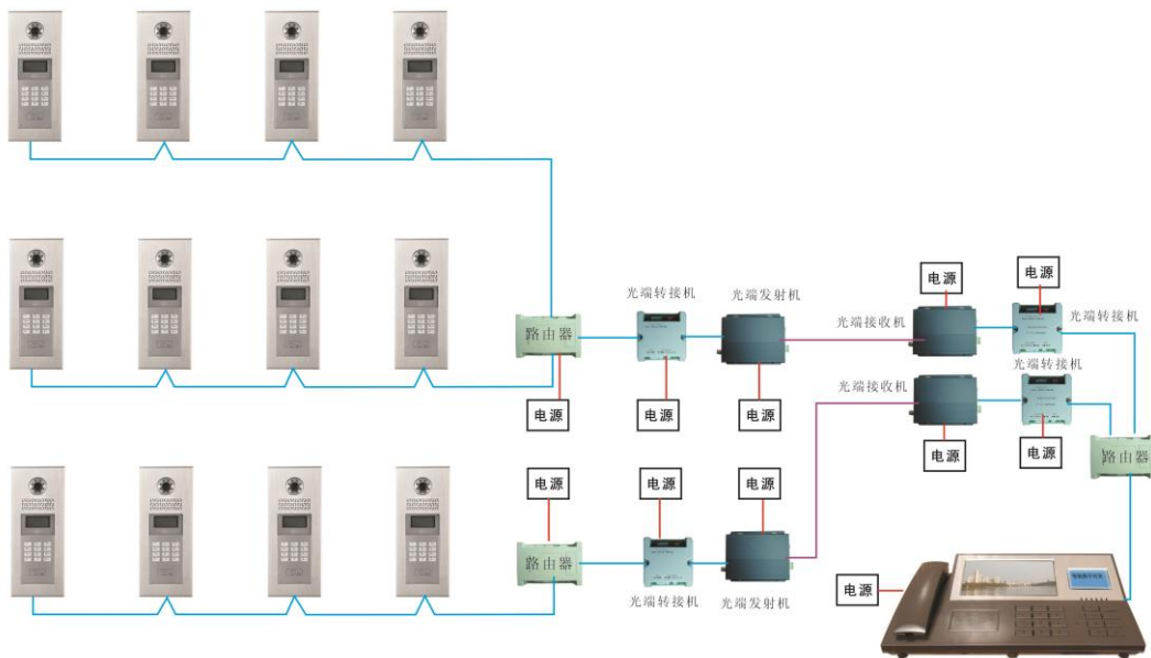
光端机连接示意图1
