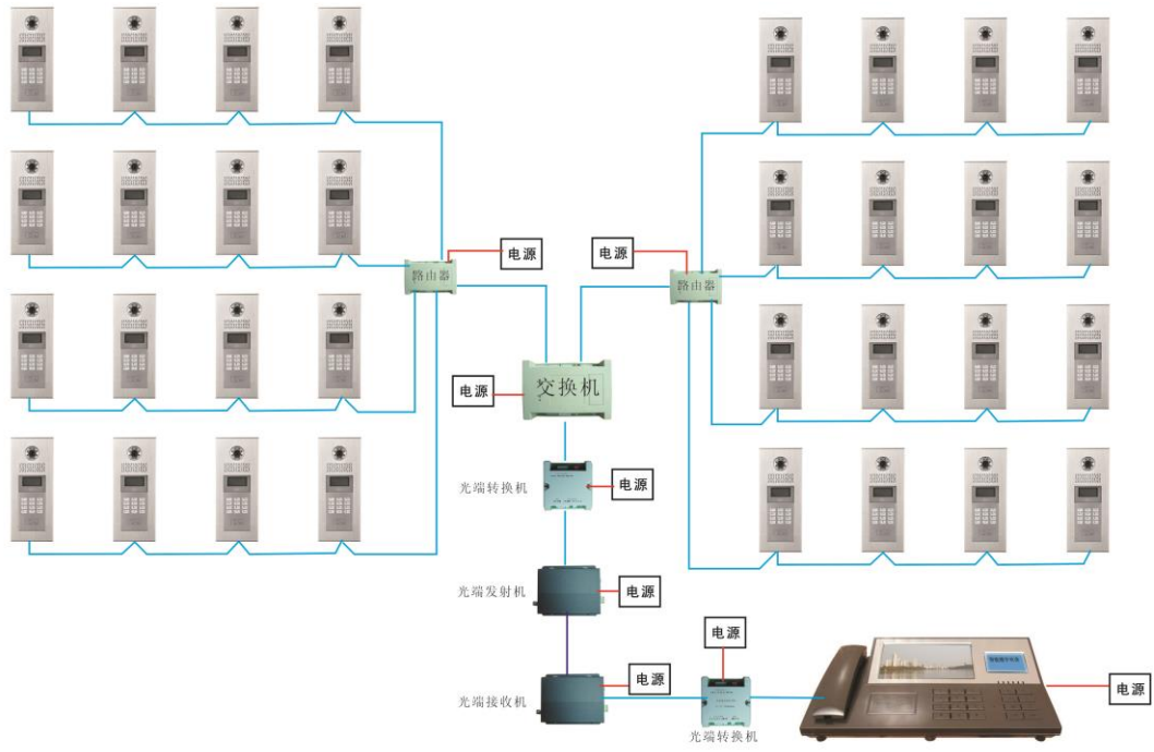
光端机连接示意图2
